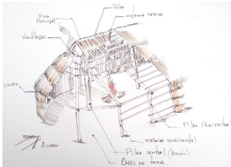
Figura5 Croquis con los elementos de una ruka.
