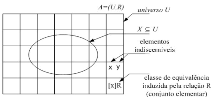
Figura 2 - Espaço aproximado A = (U, R) e X \subseteq U Fonte: Adaptado de PAWLAK, 1982; 1991.
