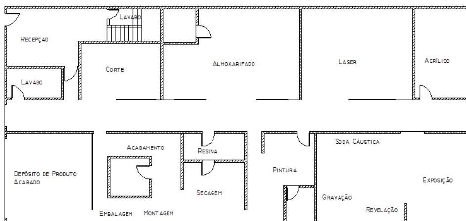
Figura 12 – Arranjo físico da Alternativa I. Fonte: O autor.
