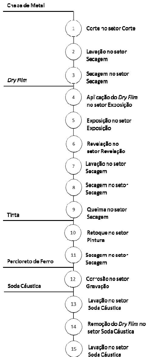
Figura 3a – Carta de Processo do Grupo 1. Fonte: O autor.
