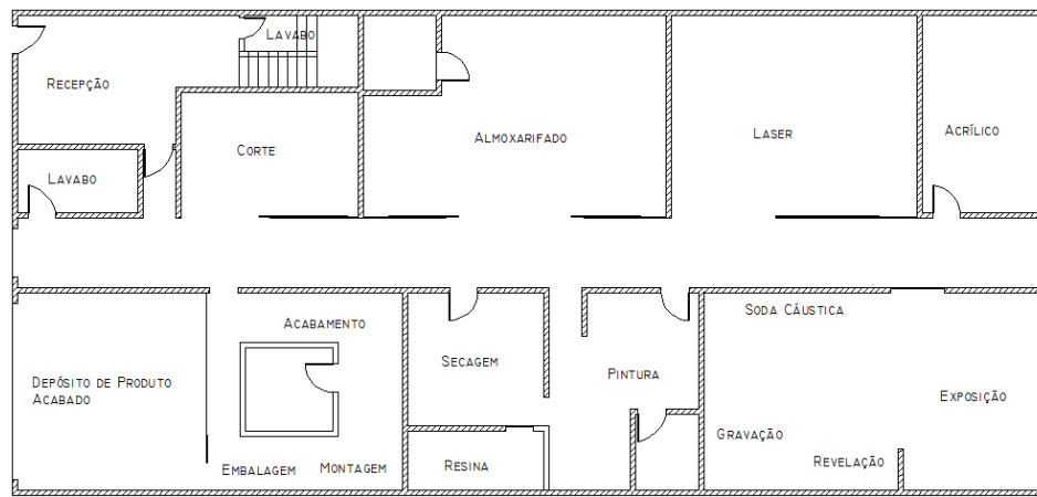
Figura 13 – Arranjo físico da Alternativa II.
