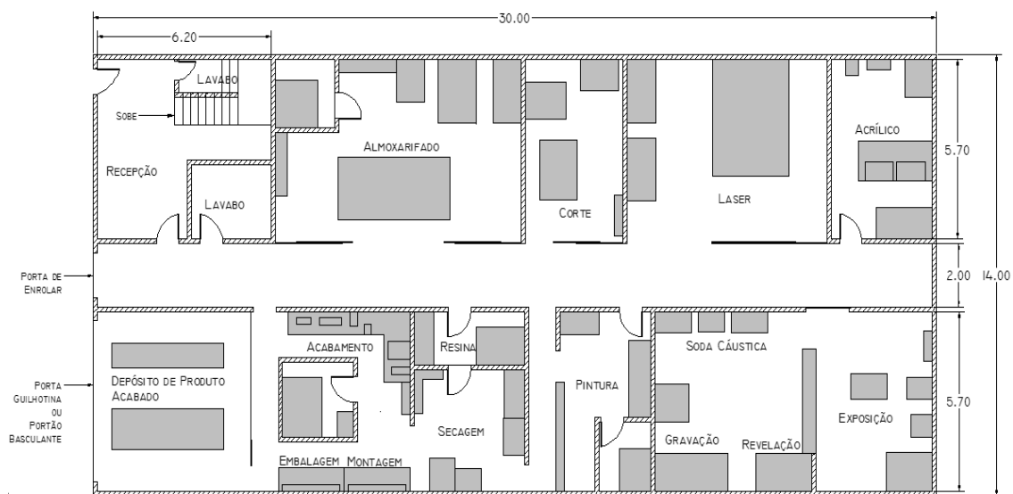
Figura 14 – Arranjo Físico Final – Térreo.
