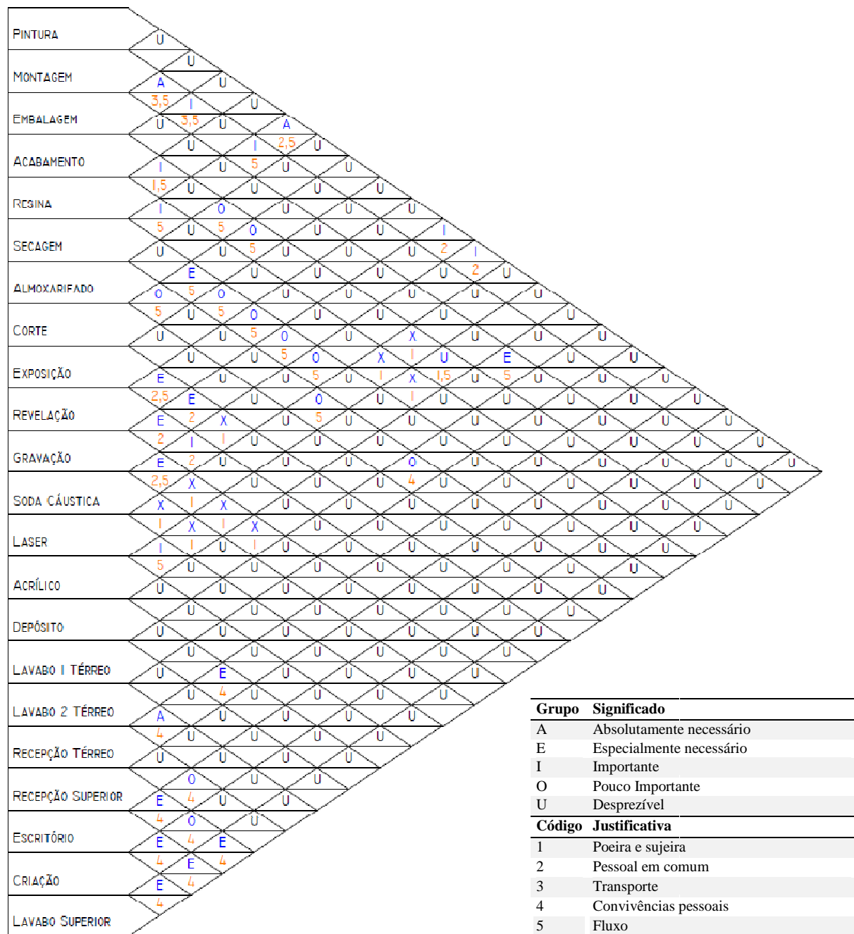
Figura 7 – Carta Fonte: O autor.
