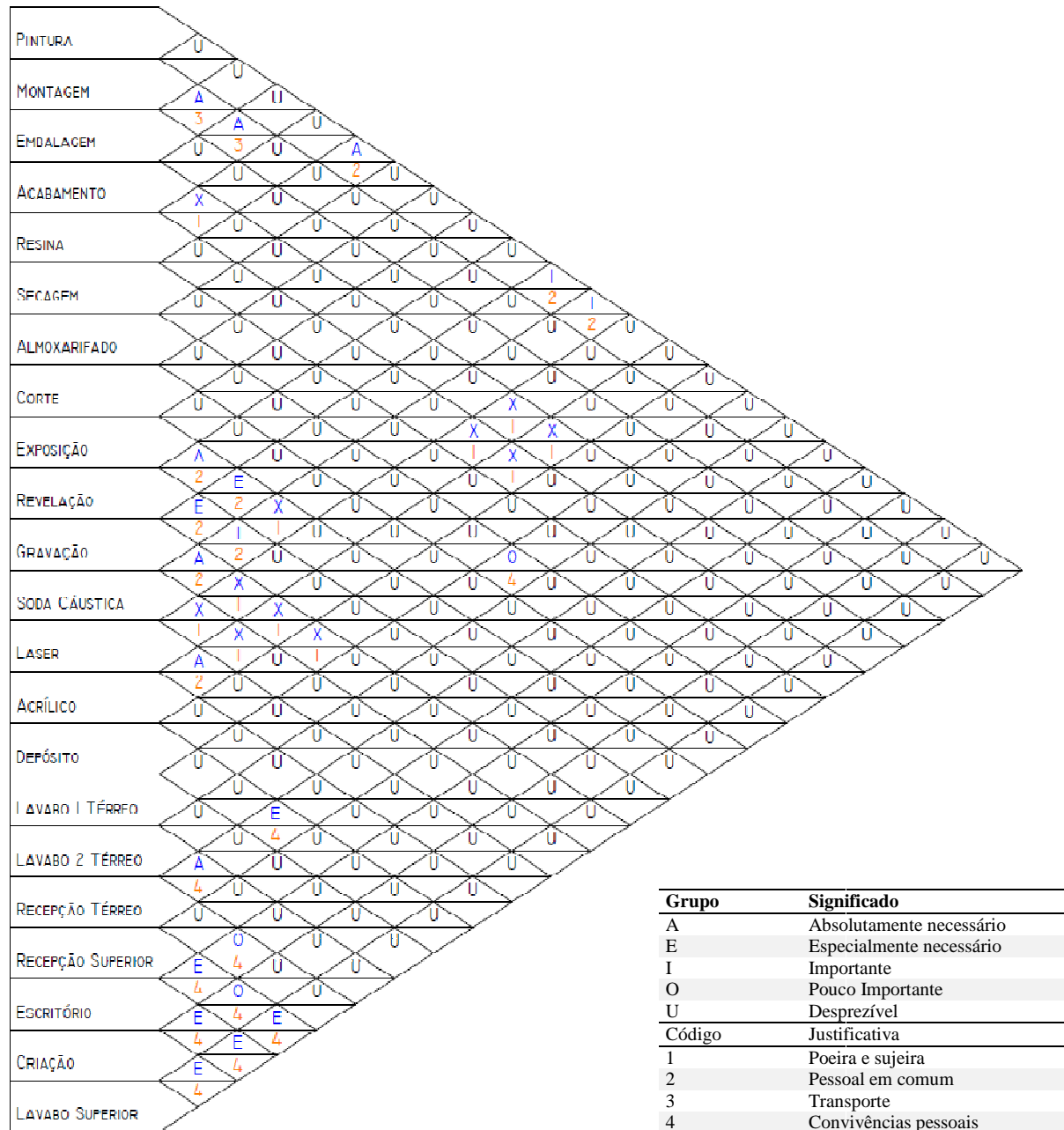
Figura 6 – Carta de Inter-relações Preferenciais. Fonte: O autor.
