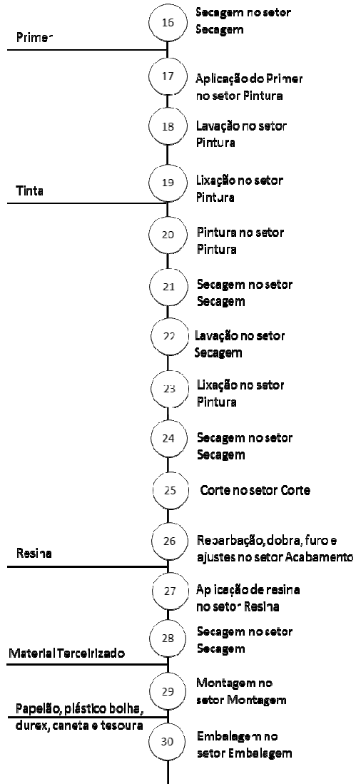
Figura 3b – Carta de Processo do Grupo 1. Fonte: O autor.
