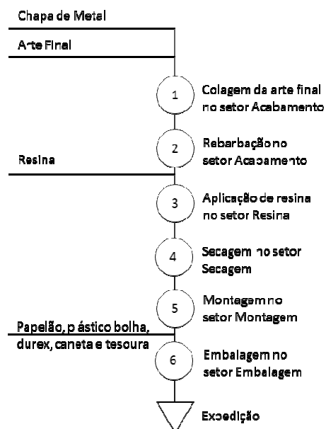
Figura 4 – Carta de Processo do Grupo 2. Fonte: O Autor
