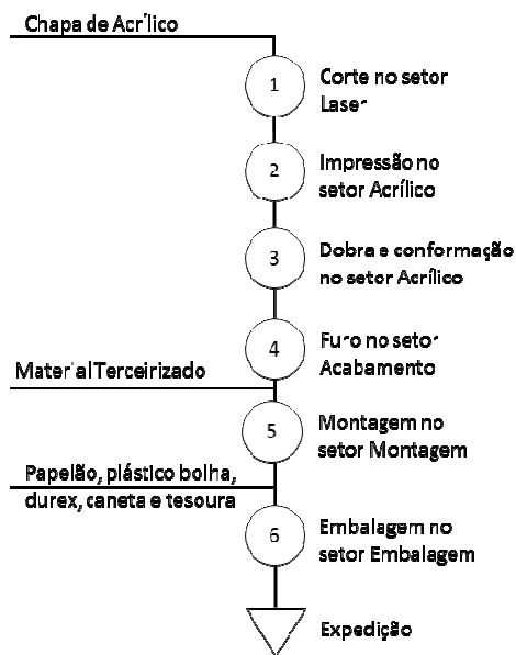
Figura 5 – Carta de Processo do Grupo 3. Fonte: O Autor
