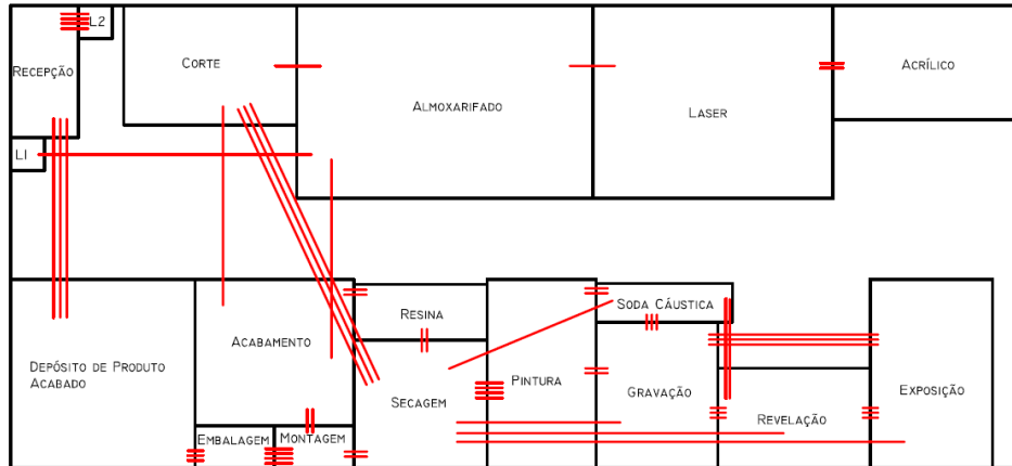
Figura 10 – Diagrama da alternativa I. Fonte: O autor.
